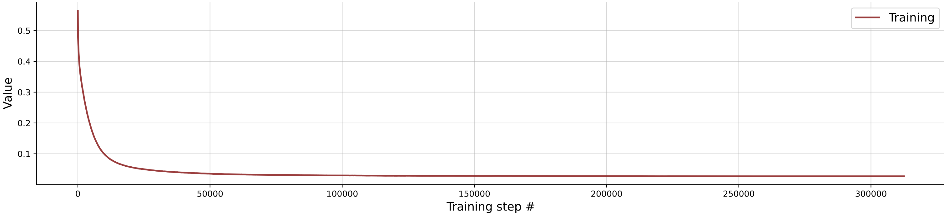
W.Decay
