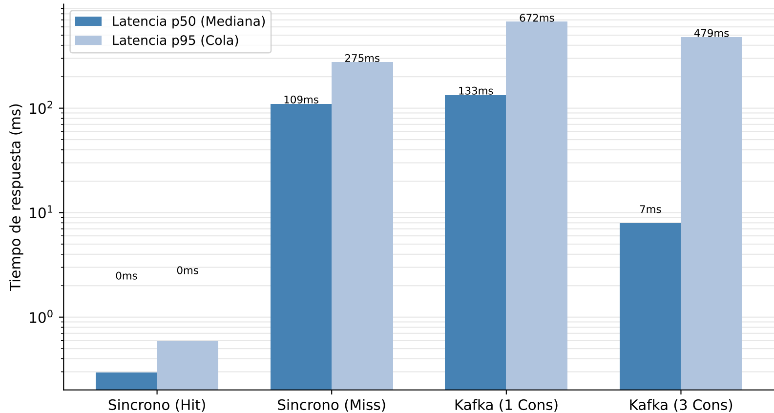
Latencias de Respuesta p50 y p95 (Escala Logaritmica)
