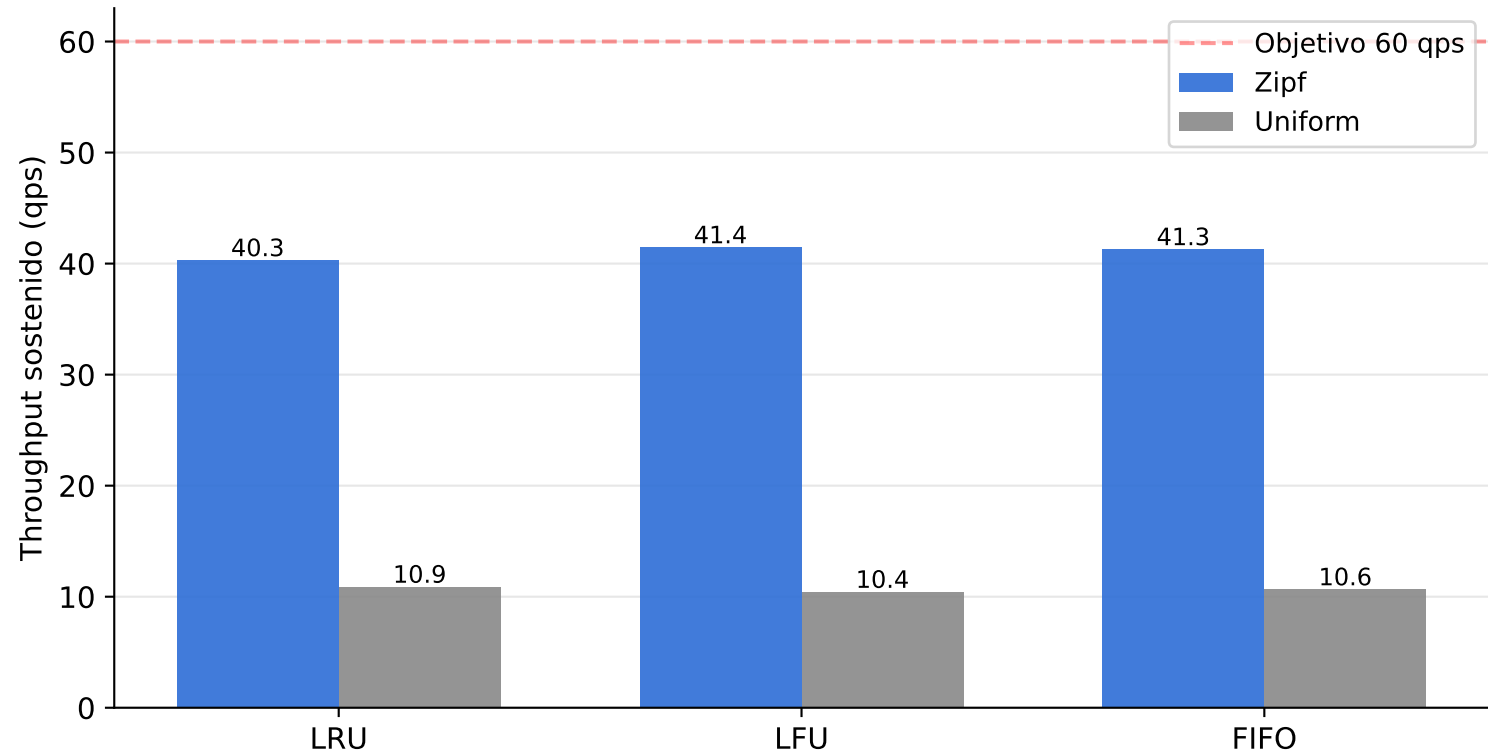
Throughput por politica y distribucion (cache 50 MB)
