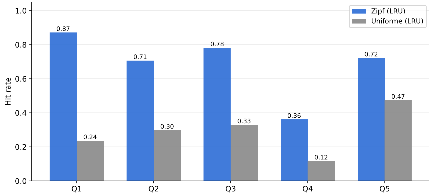
Hit rate por tipo de consulta Q1-Q5 (cache 50 MB, LRU)
