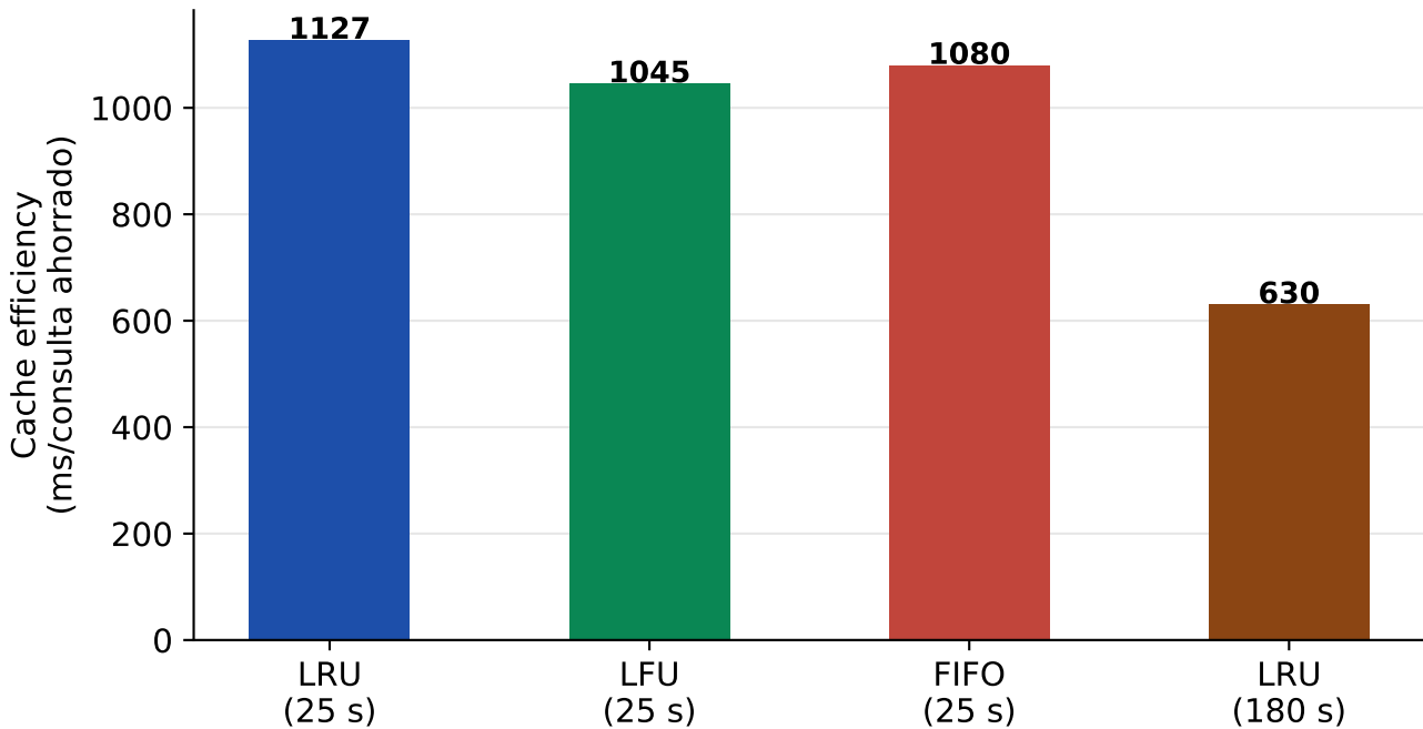
Cache efficiency por politica y duracion (Zipf, 50 MB)
