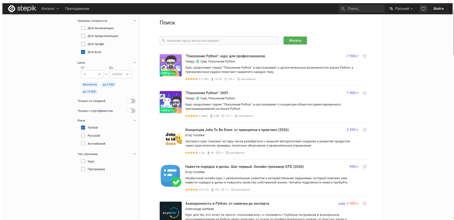
Рисунок 13 – Нажатие крестика
