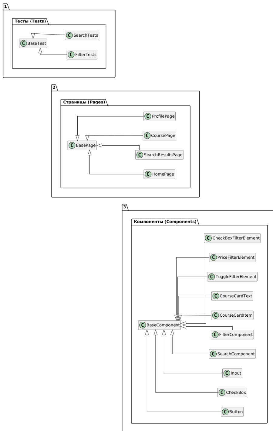
Рисунок 30 – UML-диаграмма
