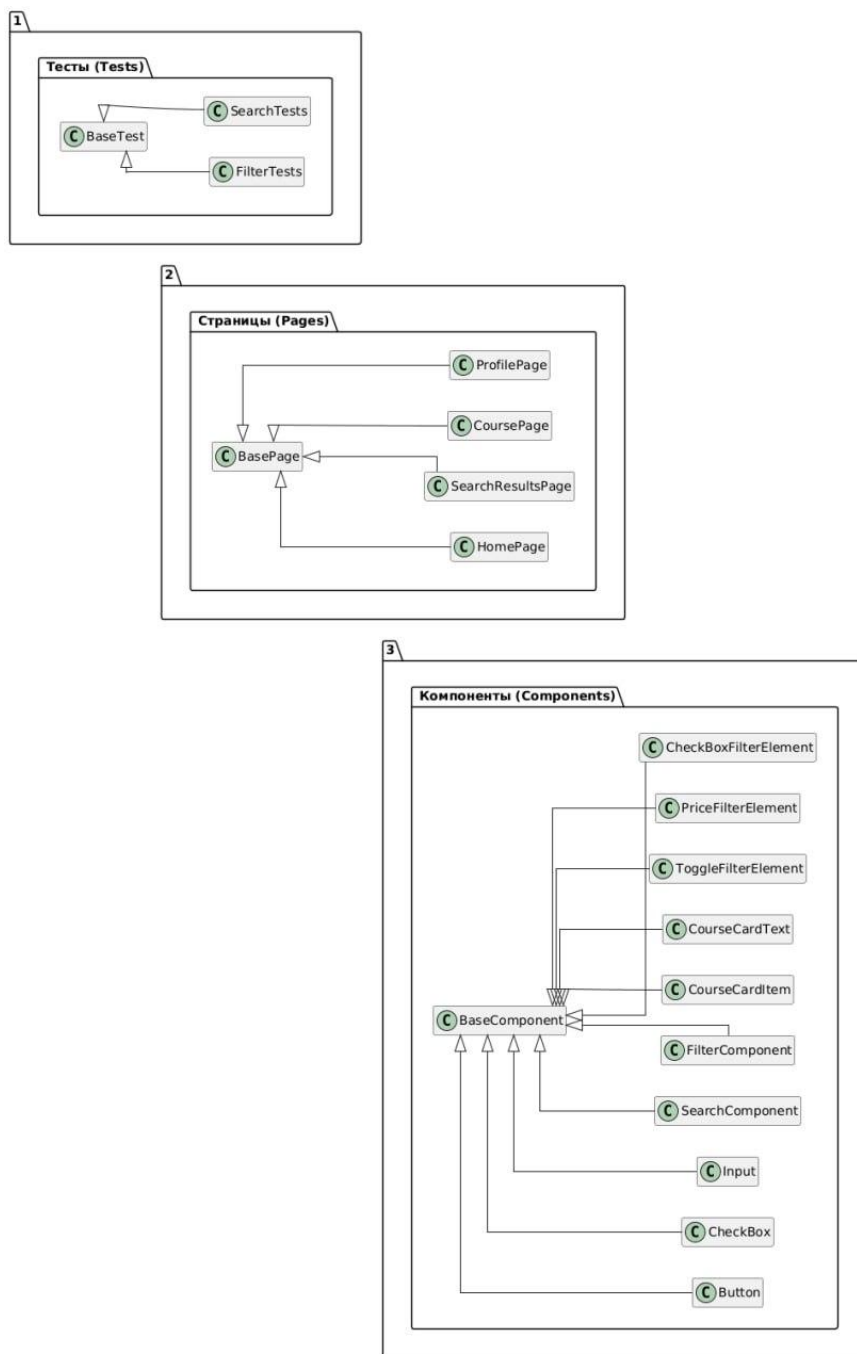
Рисунок 30 - UML-диаграмма
