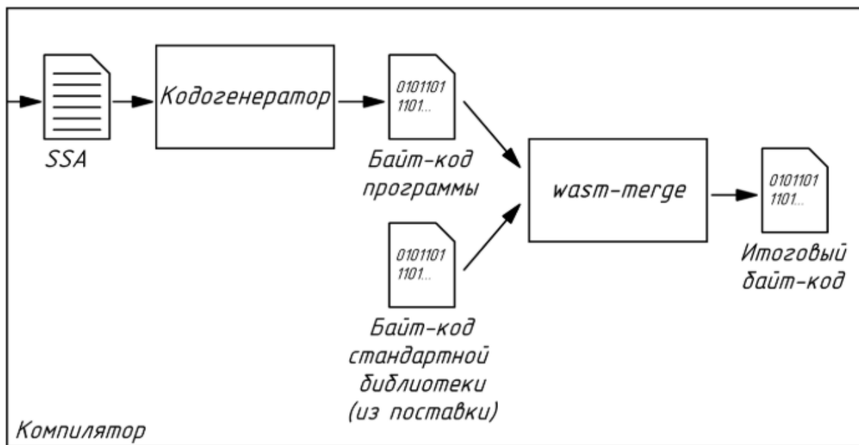
Рисунок 5 – Схема создания модуля WebAssembly
