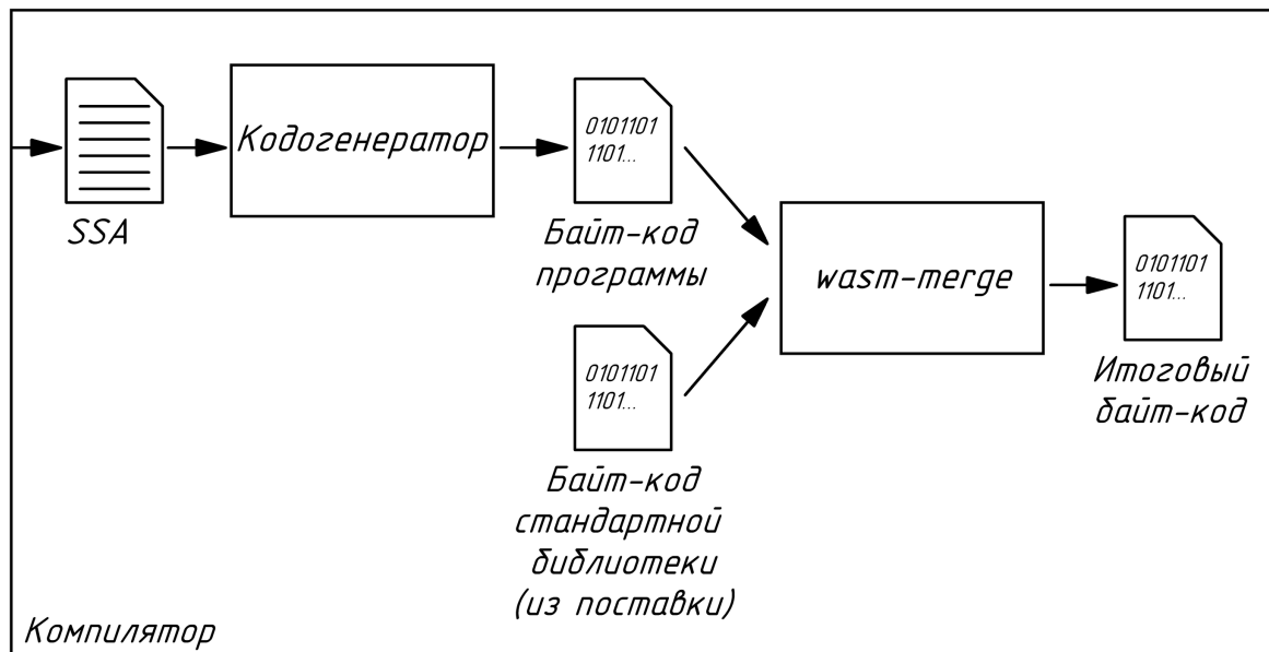
Рисунок 5 — Схема создания модуля WebAssembly
