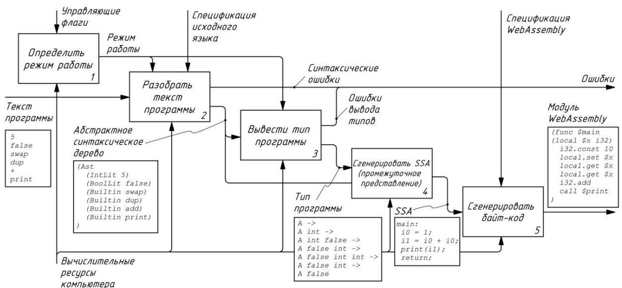
Рисунок 2 – Диаграмма декомпозиции
