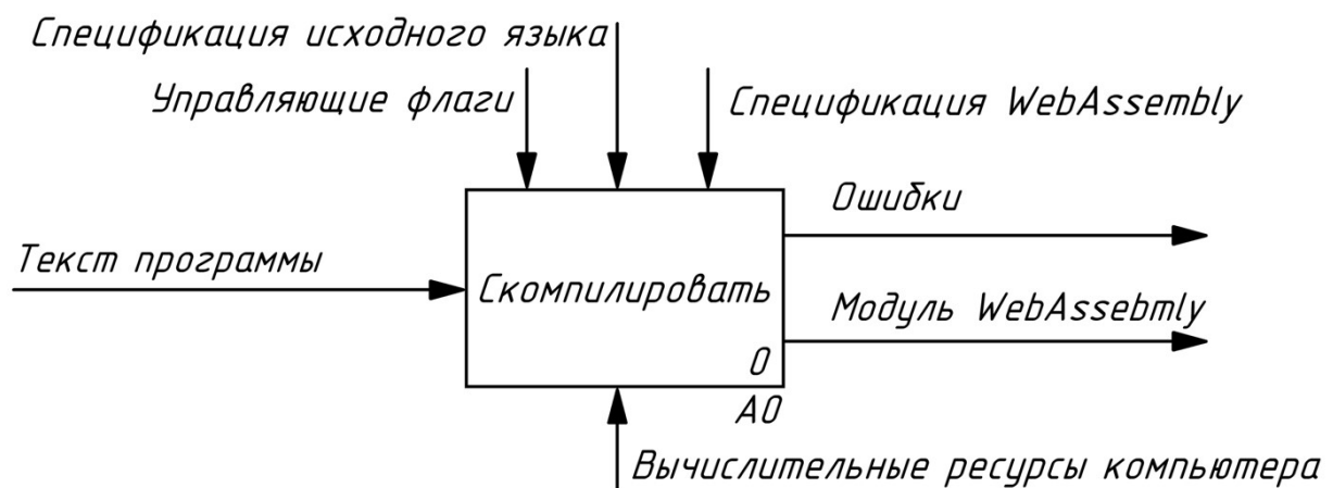
Рисунок 1 – Контекстная диаграмма
