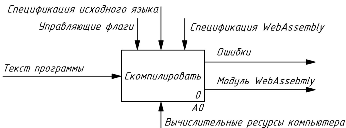
Рисунок 1 — Контекстная диаграмма
