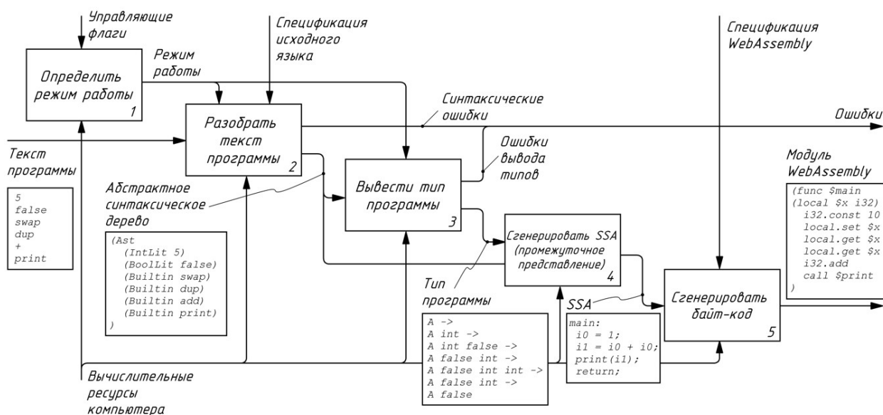
Рисунок 2 – Диаграмма декомпозиции
