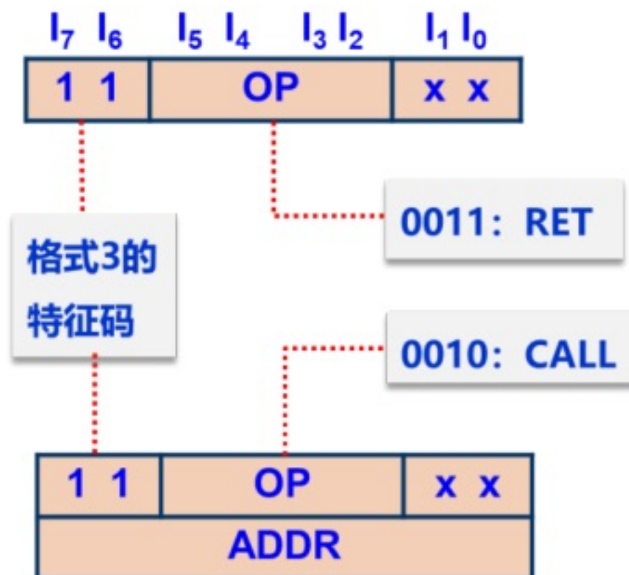
(e) 格式3: 2条过程控制指令
