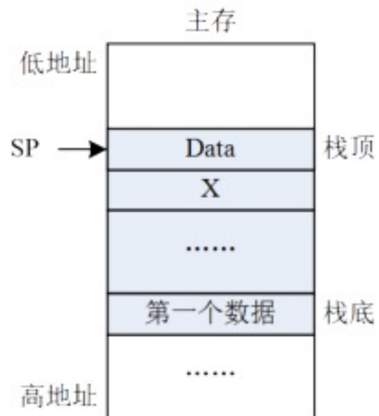
(b) PUSH R_i 后
