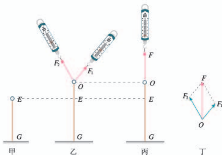
图 3.4-3 探究二力合成规律实验示意图
