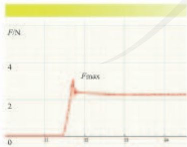
图 3.2-5 F-t 图像
