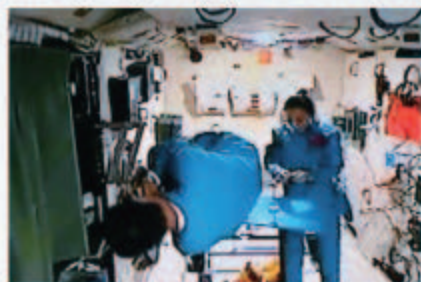
图 4.3-7 太空中质量的测量
