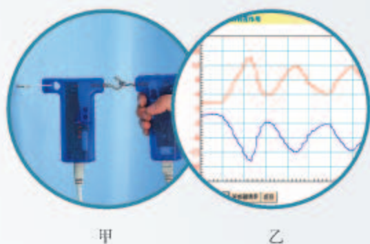
图 3.3-6 作用力和反作用力的关系
