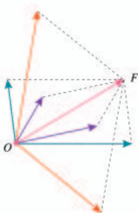
图 3.4-5 力的分解
