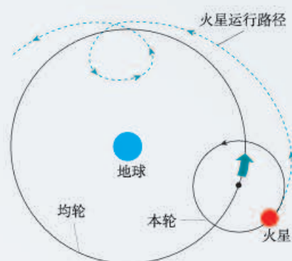
图 7.1-5 本轮和均轮
