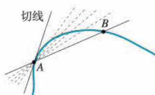
图 5.1-2 曲线的切线
