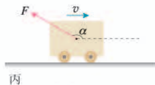
人的拉力做负功 ( \frac{\pi}{2} < \alpha \leq \pi )
