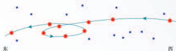
图 7.1-4 火星的逆行
