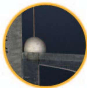
图 2.5-3 测摆线长度
