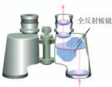
图 4.2-5 双筒望远镜中的全反射棱镜
