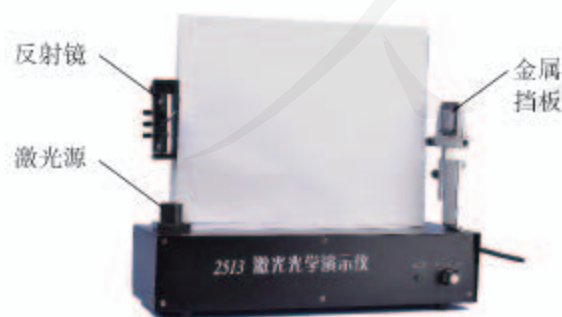
甲 实验装置(屏在挡板右侧,没有显示)
