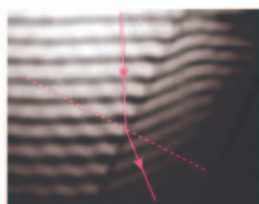
图 3.3-2 水波的折射
