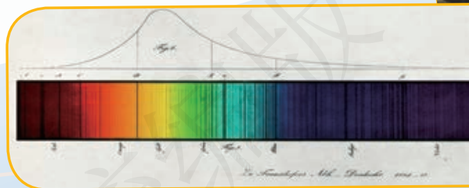
夫琅禾费线
