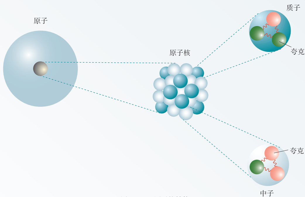
图 5.5-2 原子核结构
