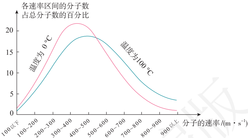
图 1.3-2 氧气分子的速率分布图像
