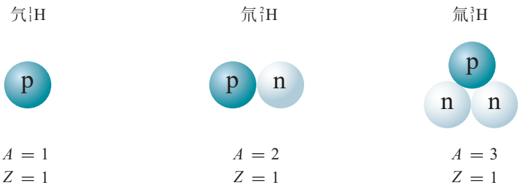
图 5.1-7 氢的同位素
