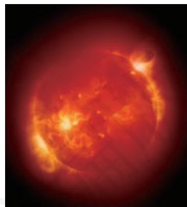
图 5.4-7 太阳
