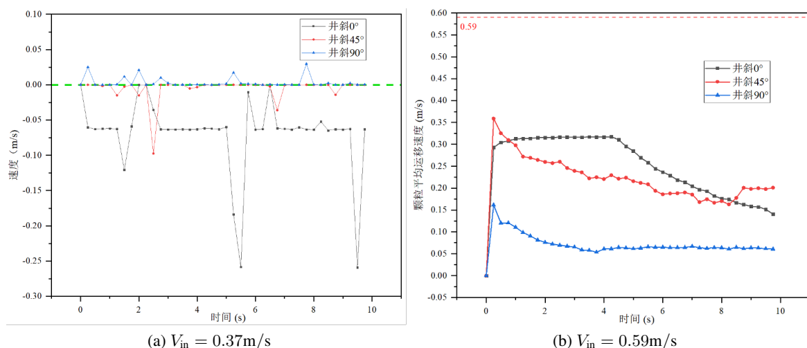
图 1.17: 钕锆垢颗粒在沉积域运移平均速度演化
