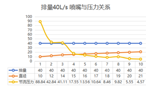
(d) 40L/s
