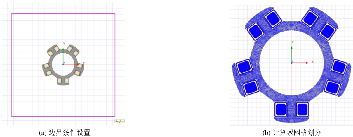
图 3.8: 上部强磁磁场分析设置
