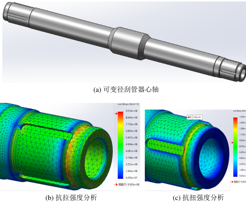
图 3.17: 可变径刮管工具薄弱零件强度有限元分析
