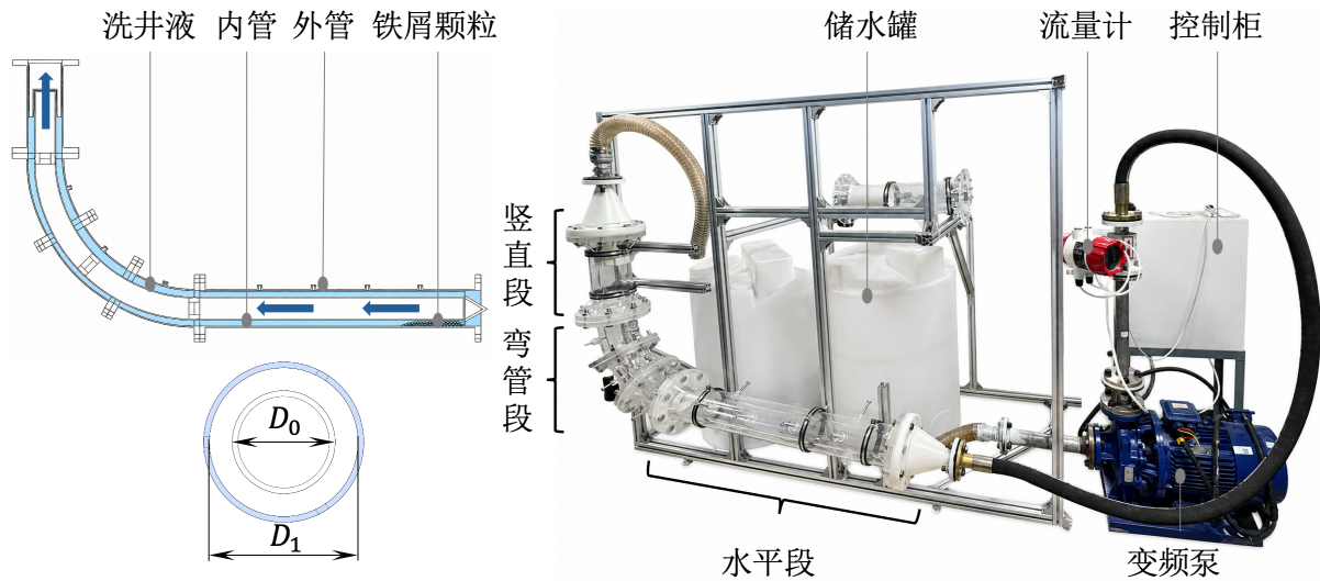
图 2.14: 研究洗井过程中铁屑运移规律的实验装置
