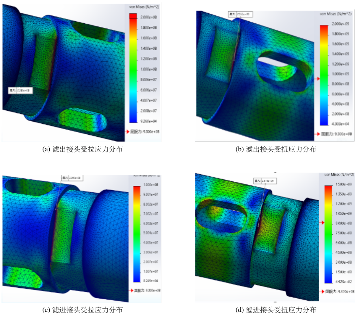
图 3.17: 过滤工具薄弱零件受载有限元分析结果
