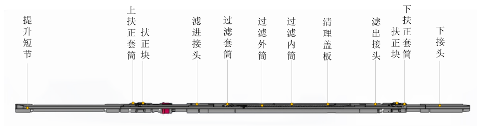
图 3.15: 多功能过滤工具结构示意图
