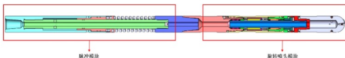
图 3.1: 水力脉冲冲砂洗井工具结构示意图
