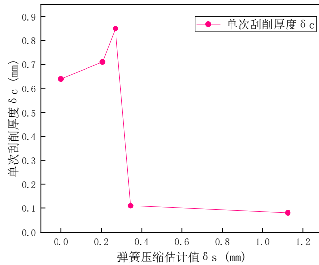
图 3.4: 刮削深度与弹簧压缩量之间的关系
