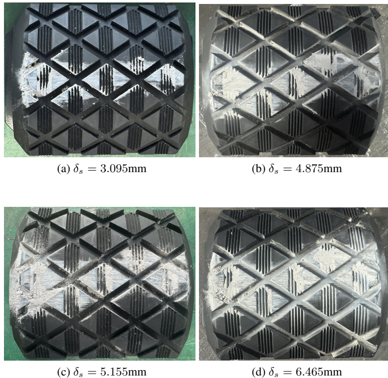
图 3.3: 刮削后刮板刀齿表面形貌及切屑堵塞情况
