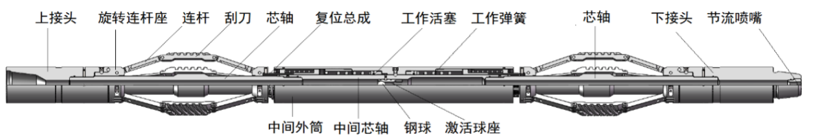
图 3.15: 可变径刮管器结构示意图
