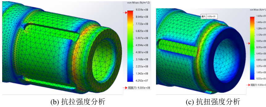
图 3.16: 可变径刮管工具薄弱零件强度有限元分析
