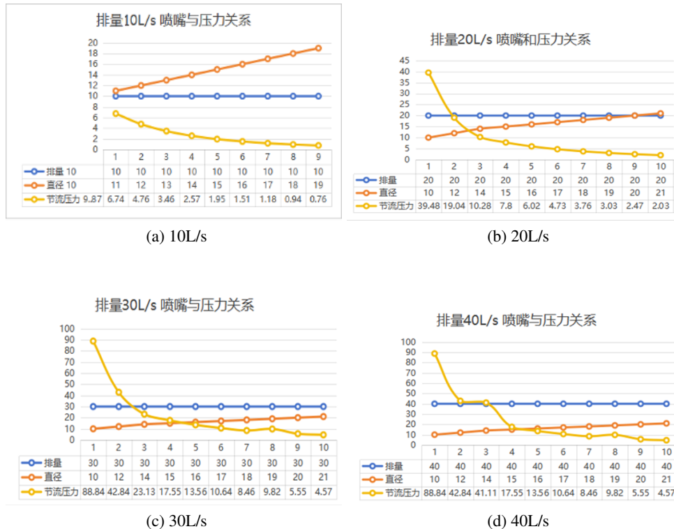
图 3.17: 喷嘴压降与排量、喷嘴尺寸之间的关系
