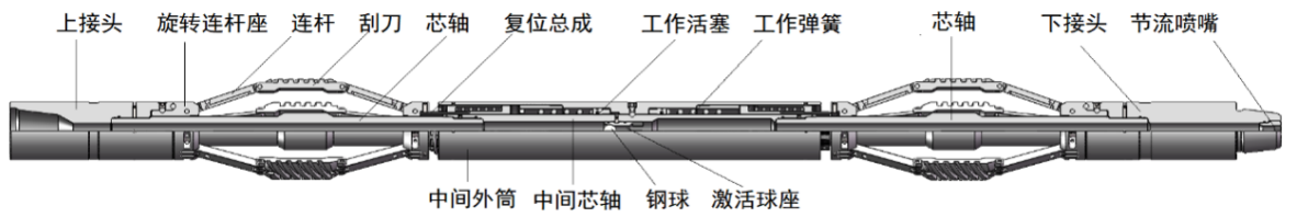
图 3.15: 可变径刮管器结构示意图
