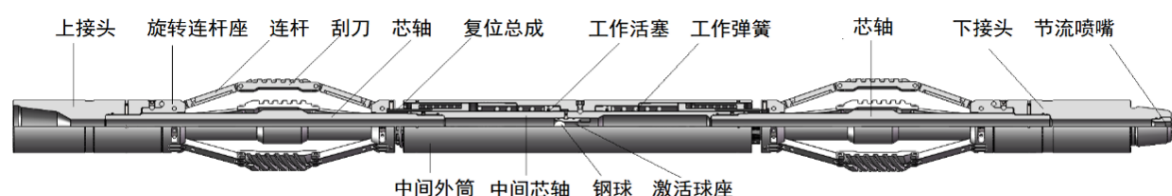
图 3.1: 可变径刮管器结构示意图
