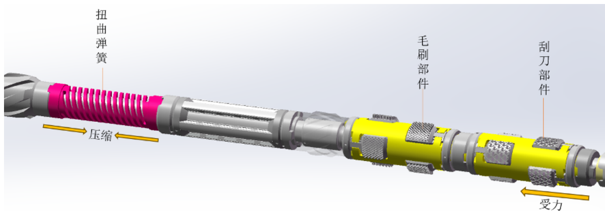
图 3.3: 弹性刮削动力系统结构
