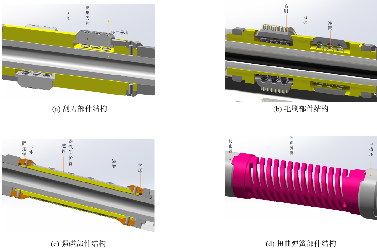
图 3.2: 四合一工具主要功能单元
