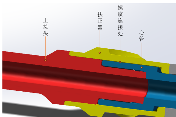
(a) 上接头结构
