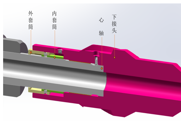
(b) 下接头结构
