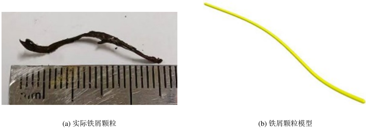
图 1.4: 铁屑颗粒及仿真模型
