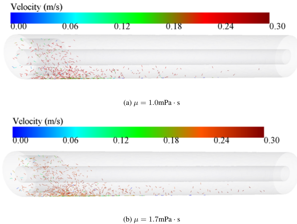
图 1.5: 压井液粘度对铁屑颗粒速度分布的影响 ( \theta = 90^\circ , v_{in} = 0.27\text{m/s} )
