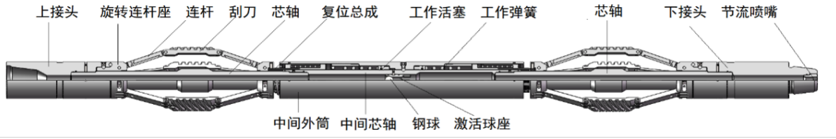
图 3.1: 可变径刮管器结构示意图
