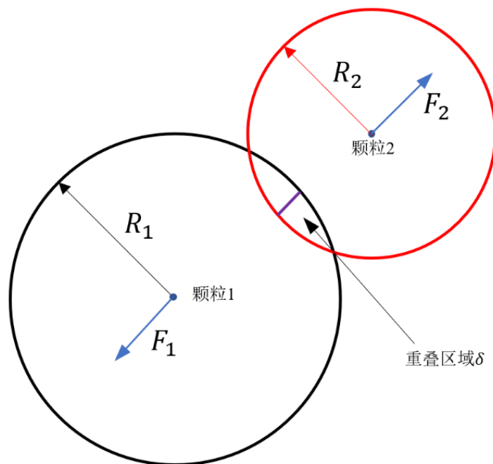
图 1.2: 双颗粒碰撞模型示意图
