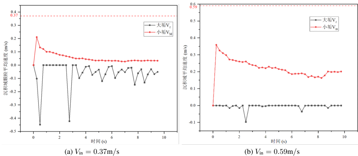
图 1.15: 钡锶垢颗粒在沉积域运移平均速度演化
