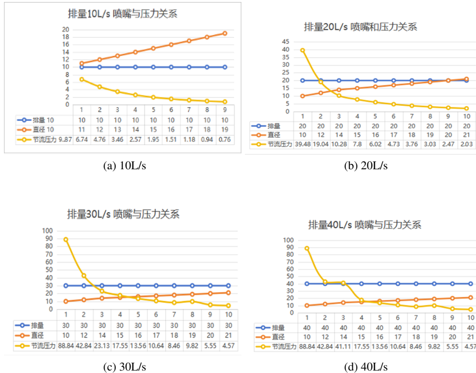
图 3.3: 喷嘴压降与排量、喷嘴尺寸之间的关系
