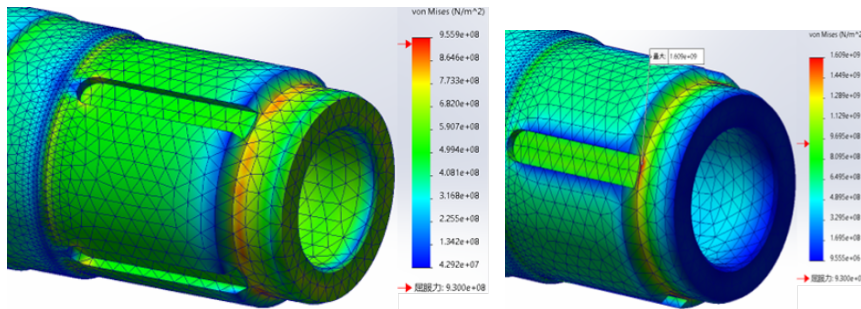
(b) 抗拉强度分析
