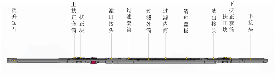
图 3.15: 多功能过滤工具结构示意图
