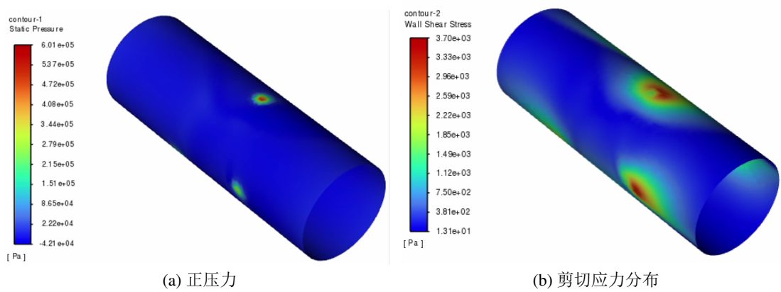
图 3.28: 水力脉冲喷头作用下套管内壁压力分布 ( t = 0.5 s)
