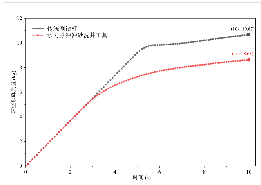
图 3.23: 环空砂砾质量变化对比图
