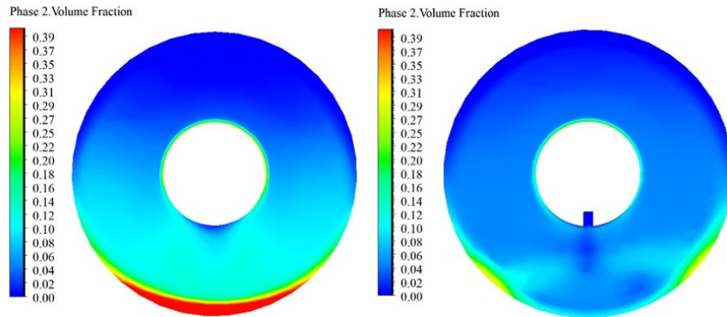
图 3.25: 喷嘴截面处砂砾体积分数对比图
