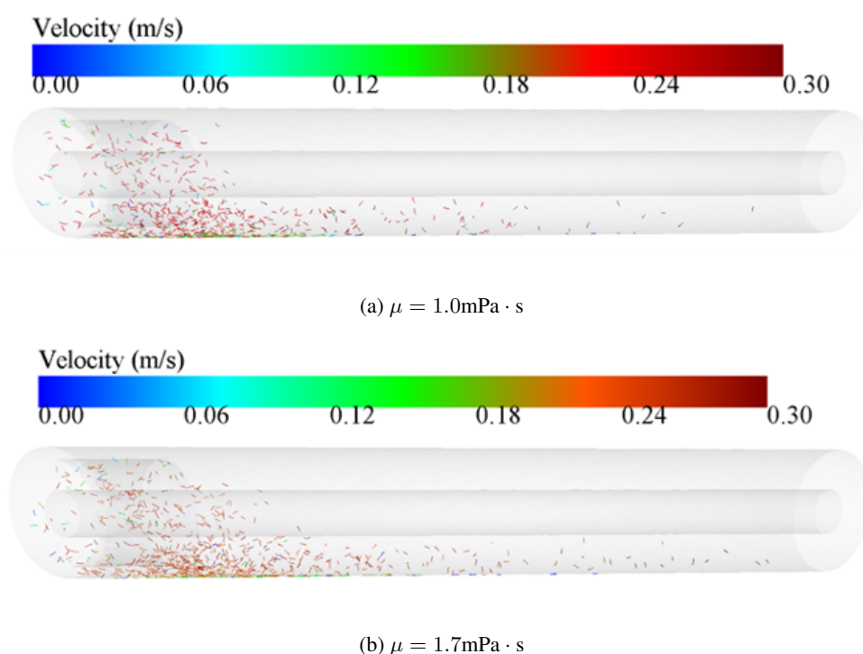
图 1.28: 洗井液粘度对铁屑颗粒速度分布的影响 ( \theta = 90^\circ , v_{in} = 0.27 \text{ m/s} )
