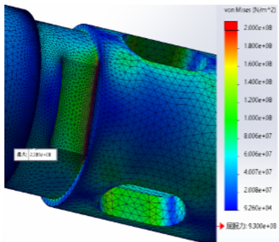
(a) 滤出接头受拉应力分布
