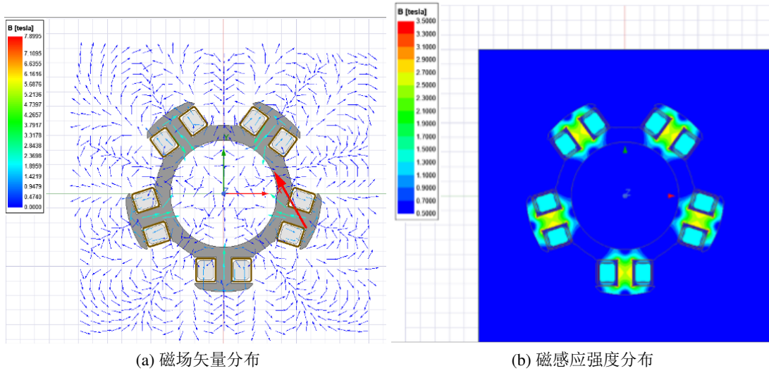
图 3.8: 磁铁径向磁化时上部强磁组件磁场计算结果
