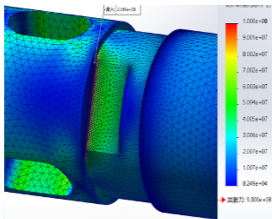
(c) 滤进接头受拉应力分布
