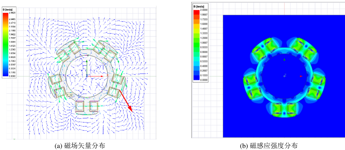
图 3.9: 磁铁周向磁化时上部强磁组件磁场计算结果
