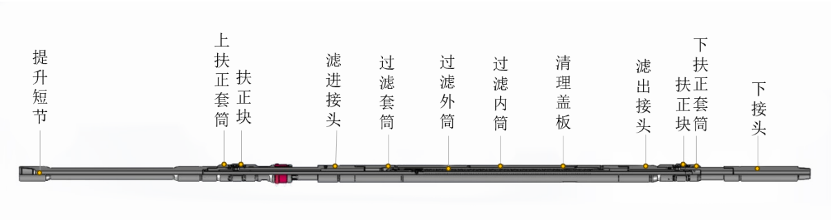
图 3.15: 多功能过滤工具结构示意图
