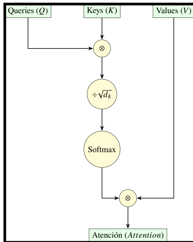
Figura 3— Mecanismo de auto-atención escalada por producto punto (Scaled Dot-Product Attention).
