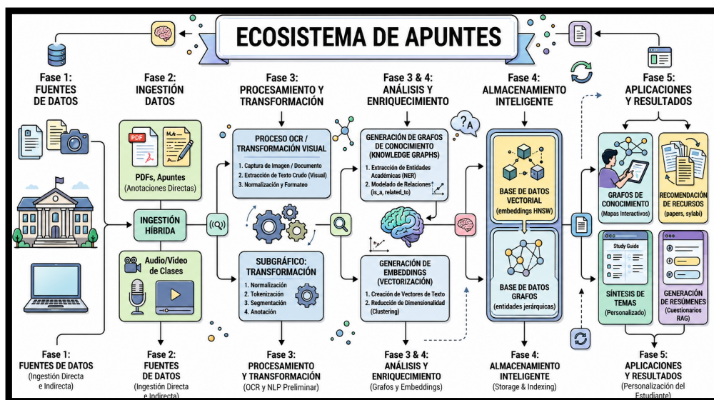
Figura 9— Pipeline adaptativo de transcripción caligráfica manuscrita (HTR) e integración RAG/Grafo en el ecosistema SynapTome.
