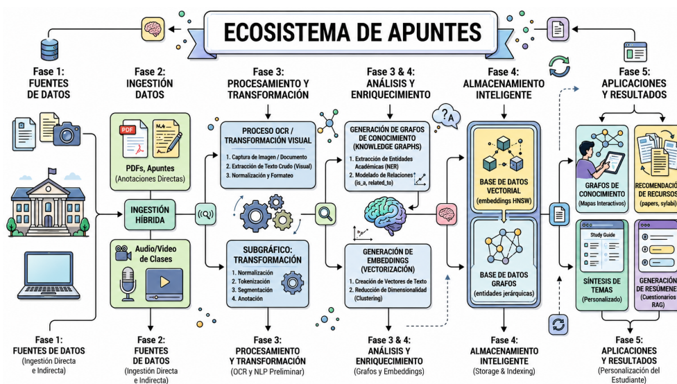
Figura 9— Pipeline adaptativo de transcripción caligráfica manuscrita (HTR) e integración RAG/Grafo en el ecosistema SynapTome.
