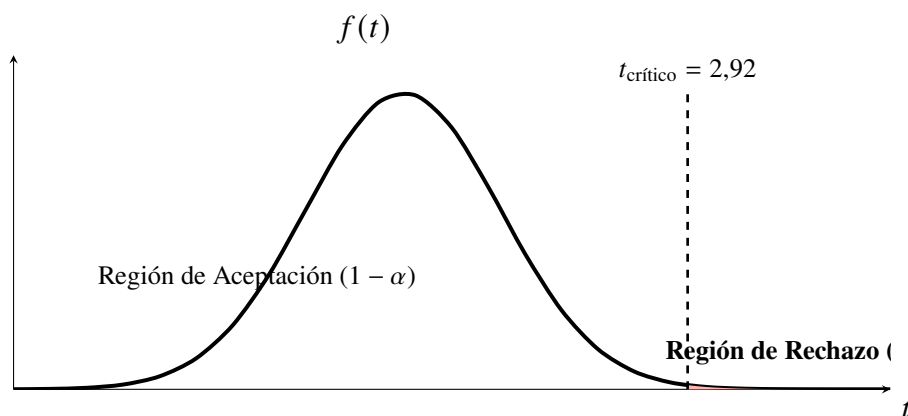
Figura 10— Representación gráfica de la curva de densidad t de Student unilateral derecha y la región crítica de rechazo.
