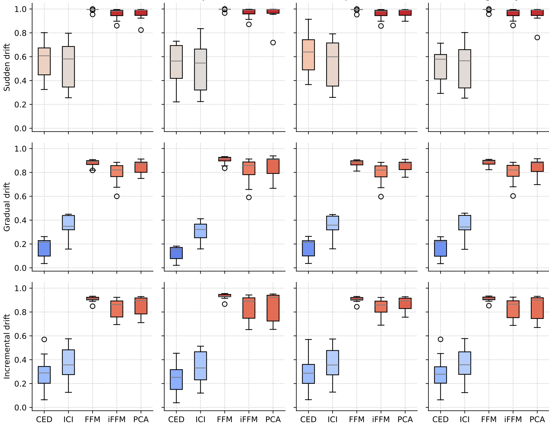
NMI
