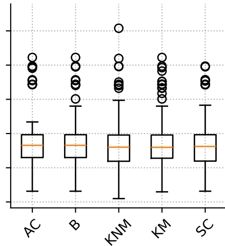
Rand
