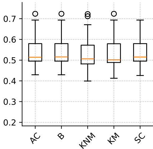
NMI
