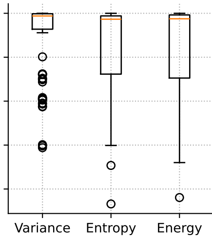
Rand
