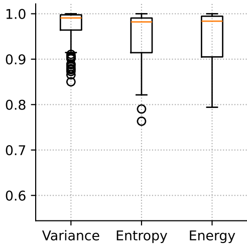
NMI
