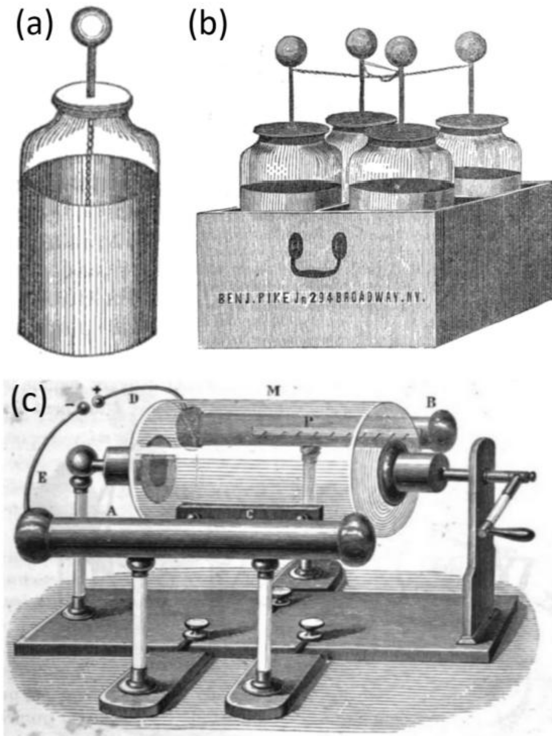
Figura 1. (a) Botella de Leyden: un recipiente de vidrio que actúa como dieléctrico, con un revestimiento interior de hojalata conectado por una cadena al terminal superior; una hoja exterior (conectada a tierra) forma la segunda armadura [19]. (b) Batería de botellas de Leyden (“batería de Franklin”) en una caja de madera [19]. (c) Máquina eléctrica de cilindro de
