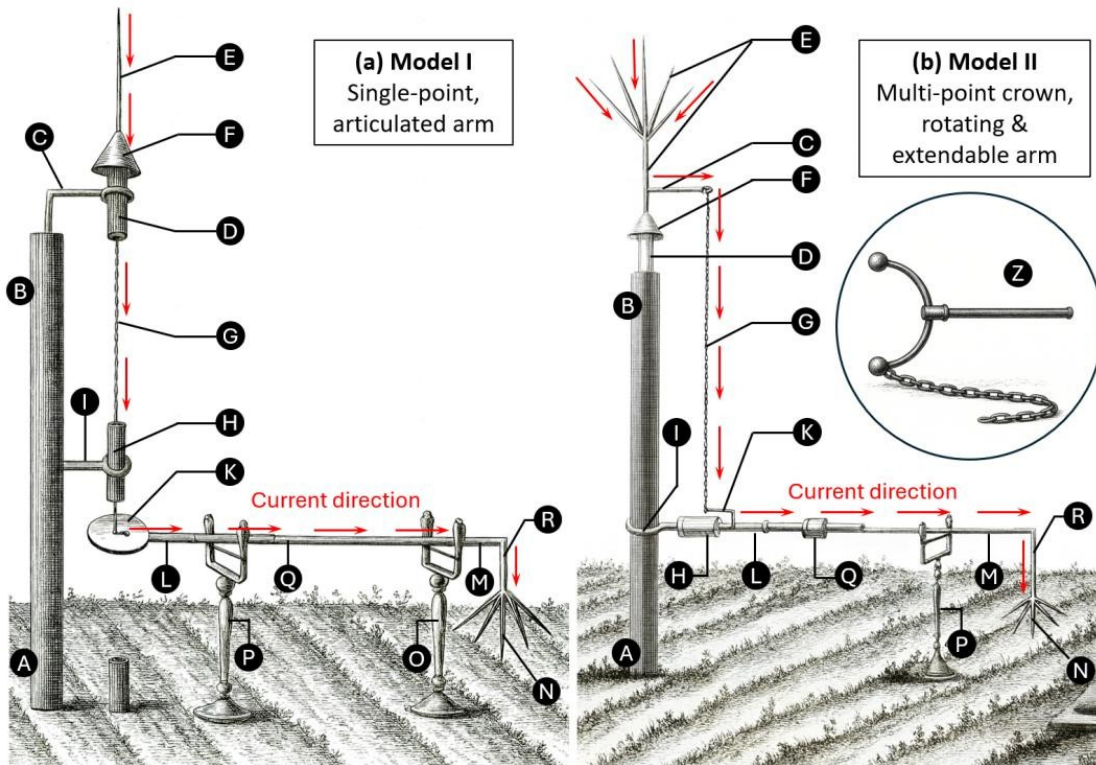
Figura 6. Electró-végétomètre de Bertholon. (a) Modelo I: colector de punto único y brazo articulado. (b) Modelo II: corona de puntos, brazo giratorio extensible. Ambos incluían un dispositivo de neutralización (Z) [31].
