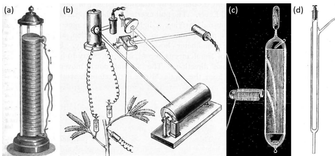
Figura 2. (a) Pila voltaica (1800): columna de discos alternos de zinc-cobre separados por arandelas empapadas en salmuera [20]. (b) Aparato de Bose para respuestas mecánicas y eléctricas simultáneas [33]. (c) Tubo de Crookes (alto vacío) que demuestra rayos catódicos [34]. (d) Primer ozonizador de Werner von Siemens (1857) [35].
