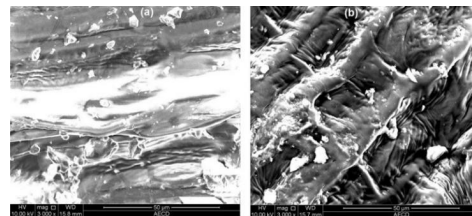
Figura 9. Imágenes SEM de superficies de semillas de trigo tratadas durante 90 s con (a) control (sin plasma), (b) plasma Ar/ \text{O}_2 . Barra de escala es 50 \mu\text{m} . Reproducido de Rahman et al., Scientific Reports , 2018, CC BY 4.0 [102].
