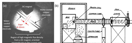
Figura 3. (a) Disco de llama Birkeland-Eyde [45]. (b) Conducto de prueba de aerosol germicida UV [48].
