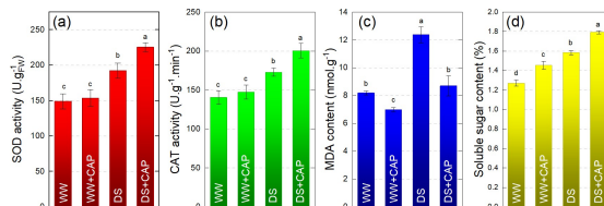
Figura 12. Efecto del estrés por sequía y el tratamiento con plasma frío sobre 4 biomarcadores en plántulas de colza: (a) actividad SOD, (b) actividad CAT, (c) contenidos de MDA, (d) contenidos de azúcares solubles. WW: bien regado; DS: estrés por sequía. Adaptado de [118].
