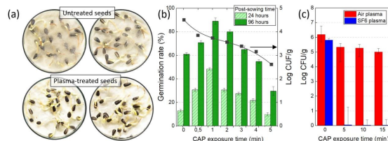
Figura 11. (a) Semillas de girasol contaminadas por Rhizopus : sin tratar vs. tratadas con plasma durante 5 min (T. Dufour, LPP). (b) Efecto del CAP sobre la germinación de Cicer arietinum y la supervivencia de microorganismos [112]. (c) Reducción de A. parasiticus en avellanas [113].
