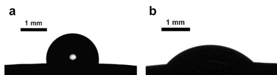
Figura 10. Gotita de agua sobre una semilla de frijol: (a) sin tratar, (b) tratada con plasma. Reproducido de Bormashenko et al., Scientific Reports , 2012, CC BY 4.0 [109].
