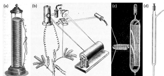
Figura 2. (a) Pila voltaica (1800): columna de discos alternos de zinc-cobre separados por arandelas empapadas en salmuera [20]. (b) Aparato de Bosc para respuestas mecánicas y eléctricas simultáneas [33]. (c) Tubo de Crookes (alto vacío) que demuestra rayos catódicos [34]. (d) Primer ozonizador de Werner von Siemens (1857) [35].
