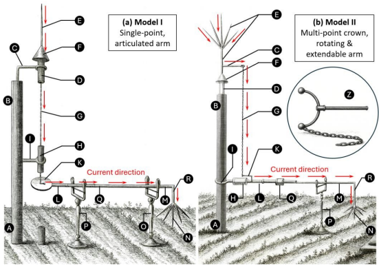
Figura 6. Electro-végétomètre de Bertholon. (a) Modelo I: colector de punto único y brazo articulado. (b) Modelo II: corona de puntos, brazo giratorio extensible. Ambos incluían un dispositivo de neutralización (Z) [31].
