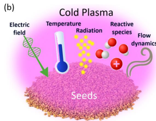
Figura 5. (a) Publicaciones anuales que contienen “agricultura plasma” (Google Scholar, 1990–2024). (b) Diagrama de semillas tratadas por CAP con sus 5 propiedades acopladas.
