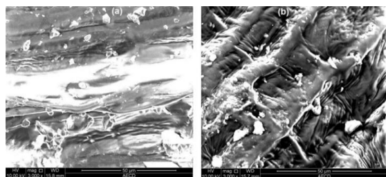
Figura 9. Imágenes SEM de superficies de semillas de trigo tratadas durante 90 s con (a) control (sin plasma), (b) plasma Ar/O 2 . Barra de escala es 50 μm. Reproducido de Rahman et al., Scientific Reports , 2018, CC BY 4.0 [102].
