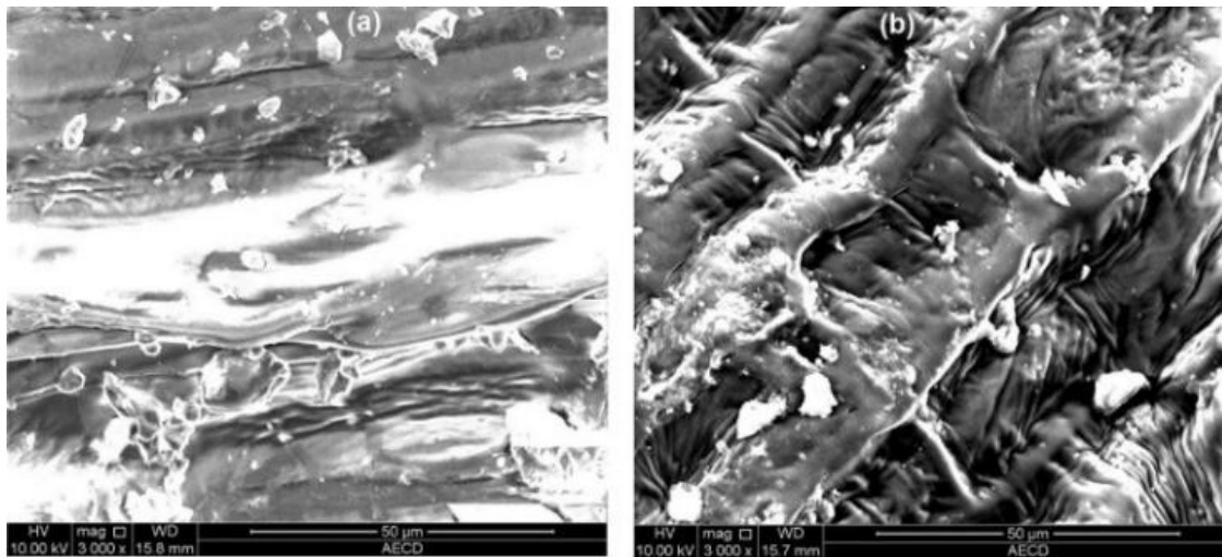
Figura 9. Imágenes SEM de superficies de semillas de trigo tratadas durante 90 s con (a) control (sin plasma), (b) plasma Ar/O 2 . Barra de escala es 50 µm. Reproducido de Rahman et al., Scientific Reports , 2018, CC BY 4.0 [102].
