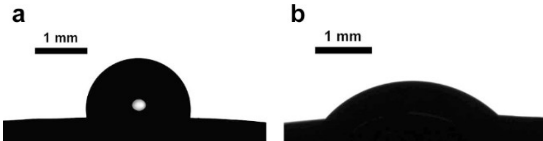
Figura 10. Gotita de agua sobre una semilla de frijol: (a) sin tratar, (b) tratada con plasma. Reproducido de Bormashenko et al., Scientific Reports , 2012, CC BY 4.0 [109].
