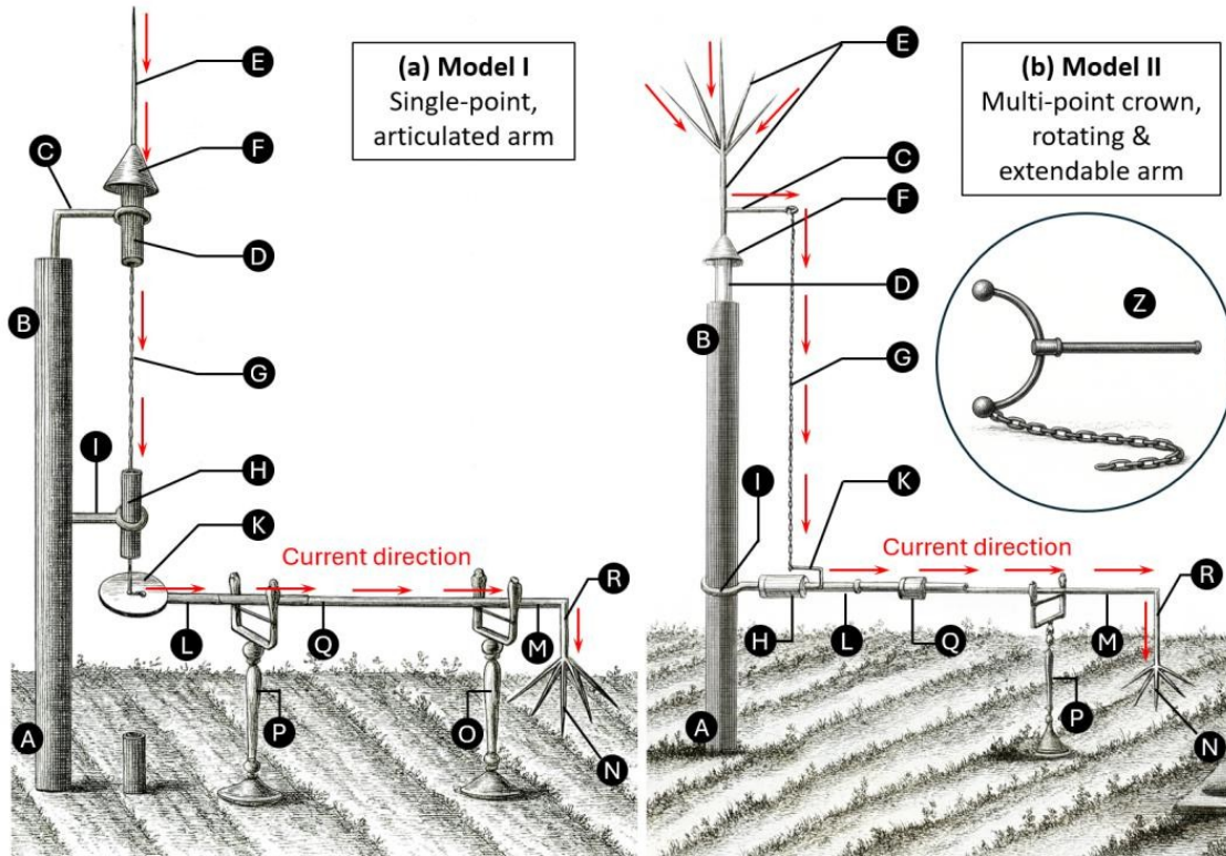
Figura 6. Electrô-végétomètre de Bertholon. (a) Modelo I: colector de punto único y brazo articulado. (b) Modelo II: corona de puntos, brazo giratorio extensible. Ambos incluían un dispositivo de neutralización (Z) [31].
