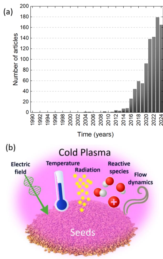
Figura 5. (a) Publicaciones anuales que contienen “agricultura plasma” (Google Scholar, 1990–2024). (b) Diagrama de semillas tratadas por CAP con sus 5 propiedades acopladas.
