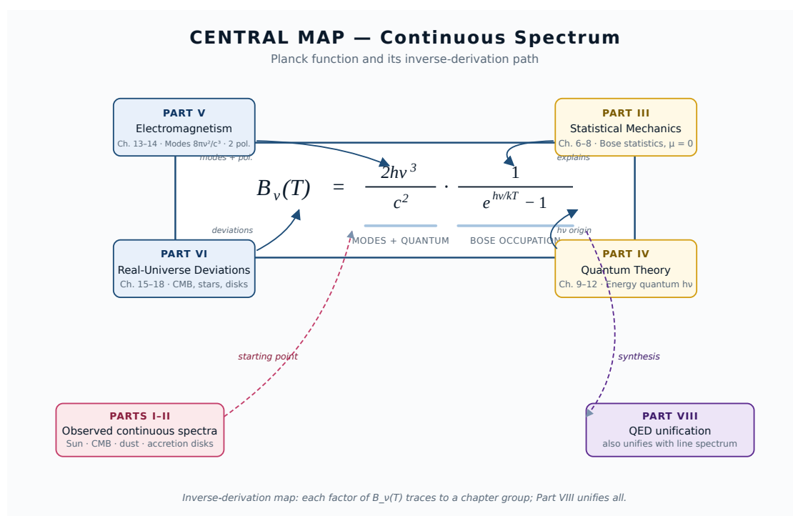
図 1: プランク関数 B_\nu(T) の各因子と、それを解き明かす章群の対応。第III部が占有因子、第IV部がエネルギー量子 h\nu 、第V部がモード密度＋偏光自由度、第VI部が現実の天体での「ずれ」を担当する。第I-II 部が観測の入口、第VIII 部が QED による統一の出口にあたる。
