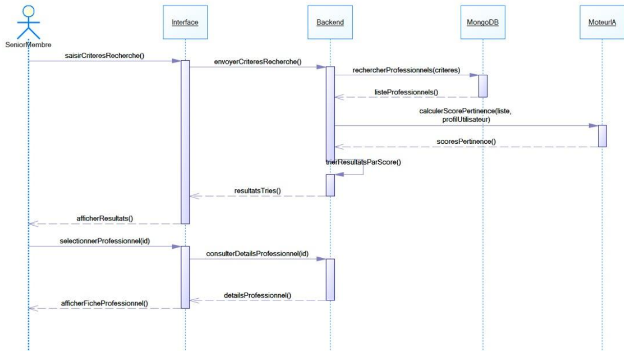
Figure 1: Diagramme de Séquence Recherche annuaire avec recommandation IA
