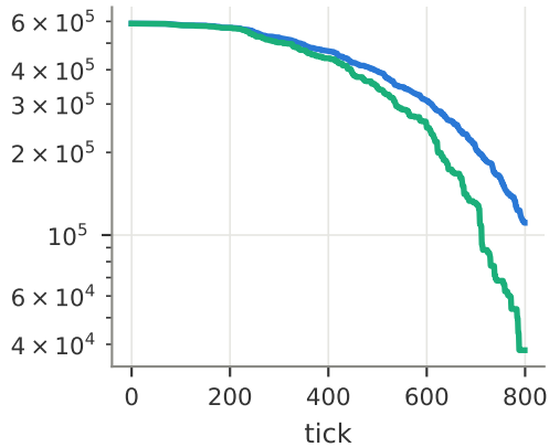
poisson 3 clusters
