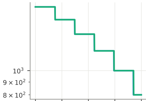
poisson 3 clusters
