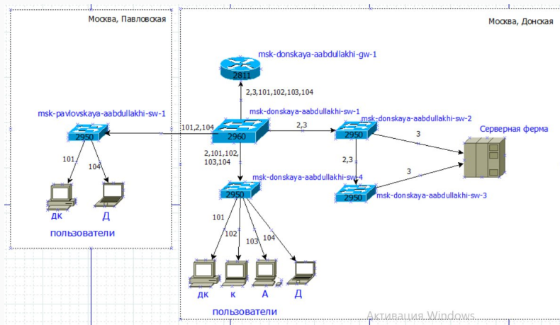
Рис. 2: Схема L2 — распределение VLAN
