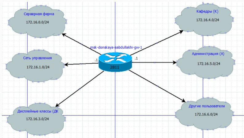
Рис. 4: адресный план для 172.16.0.0/12
