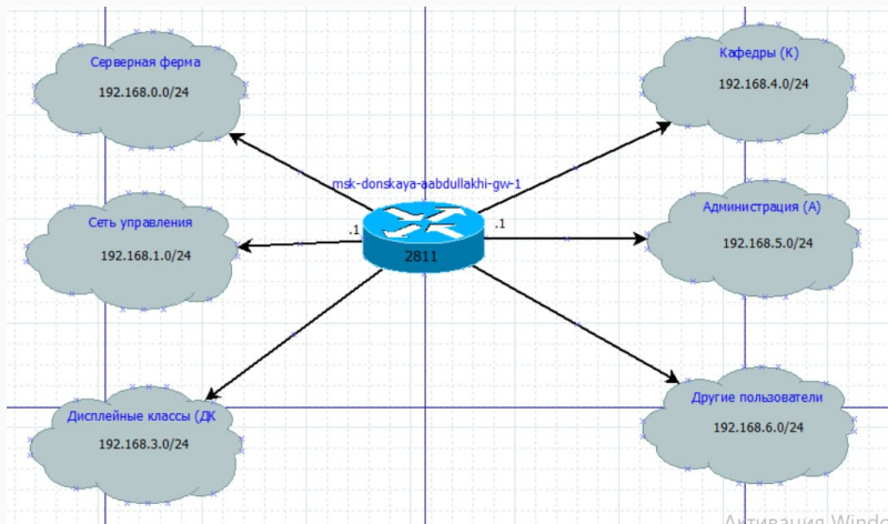
Рис. 5: адресный план для 192.168.0.0/16
