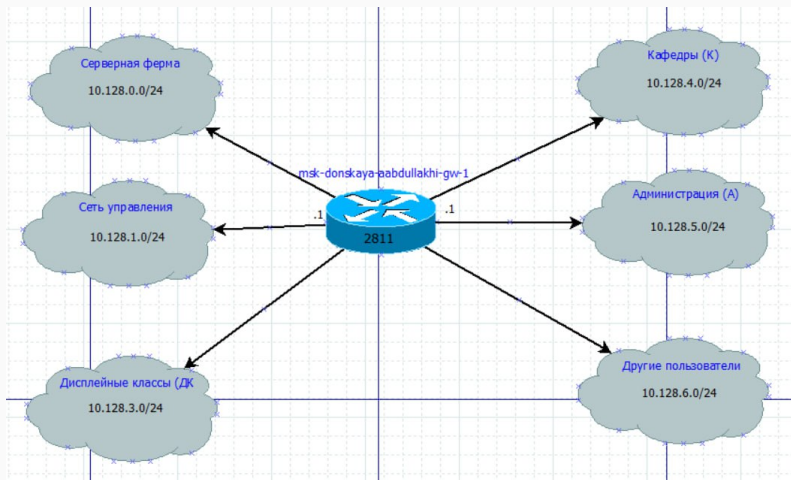
Рис. 3: Схема L3 — IP-план сети
