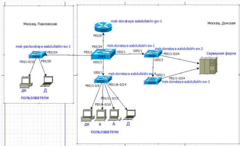
Рис. 1: Схема L1 — физическая топология
