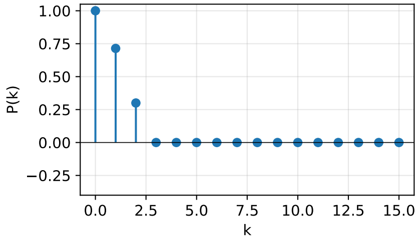
PACF (coupe après k=2)
