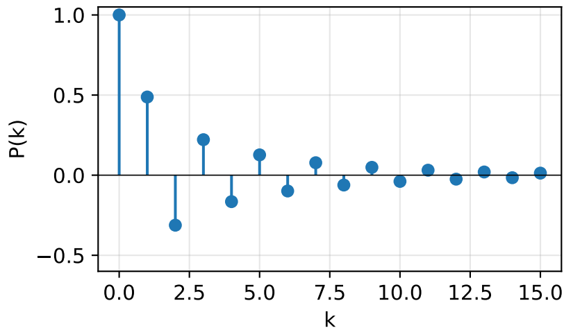
PACF (décroît)
