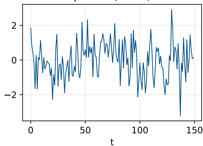
\phi = 0.3 (faible)
