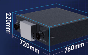
FV-15ZDP2C 新家用薄型全热交换器
