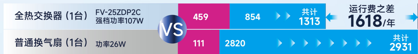
松下普通换气扇与全热交换器长期成本比较图
