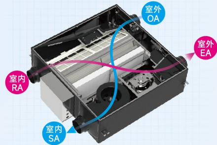
热交换模式风路图（俯视视角）
