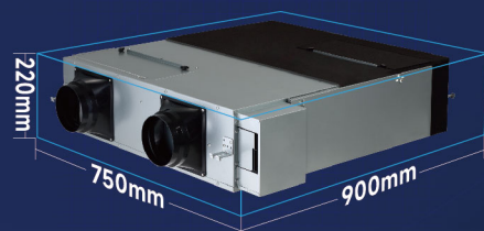
FY-15ZDP1C 家用薄型全热交换器
